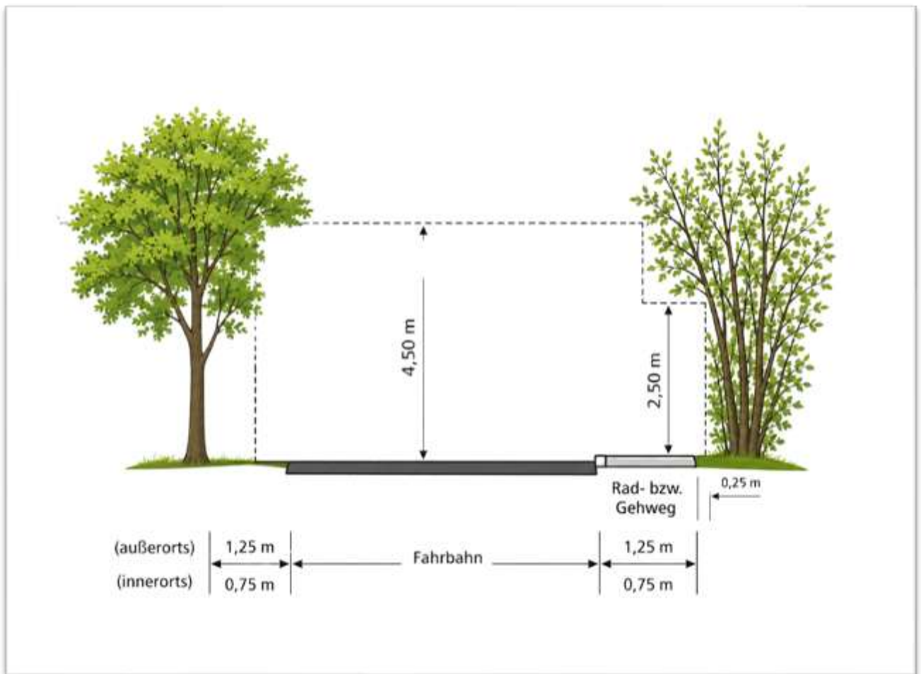
Abbildung: Skizze Lichtraumprofil
