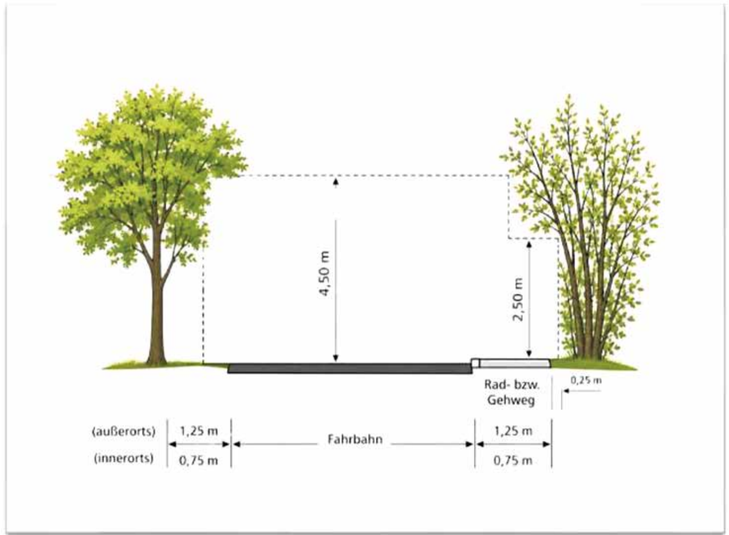
Abbildung: Skizze Lichtraumprofil
